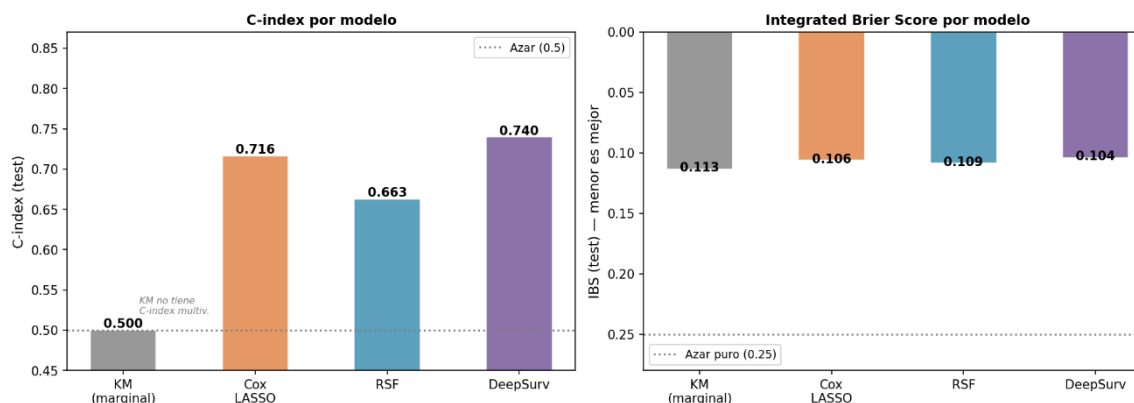
Comparativa final de rendimiento — KM / Cox-LASSO / RSF / DeepSurv | MSK_NSLC
